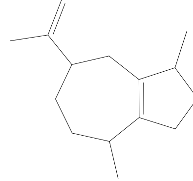
\alpha - guajen
